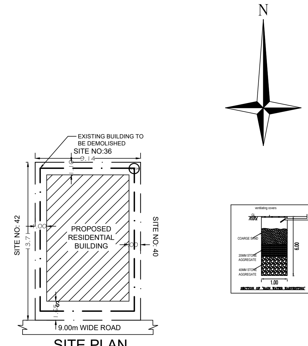
SITE PLAN 1:200
